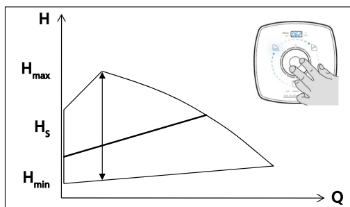
Obr. 20: Nastavení Proporcionální regulace tlaku
