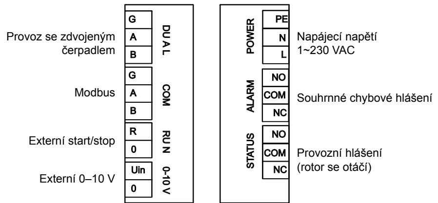
Obr. 36: Schéma elektrického zapojení typů Calio Z 40-120/-180, 50-100/-120 a 65-80/-120
