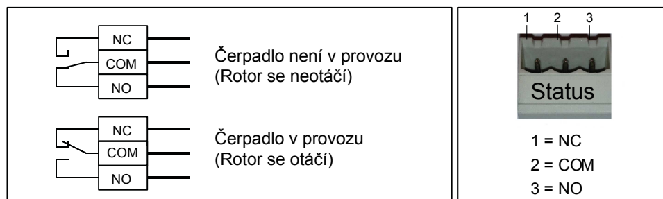
Obr. 34: Schéma zapojení: provozní hlášení
