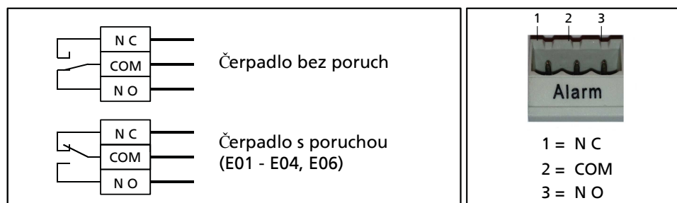
Obr. 33: Schéma zapojení: alarmové hlášení
