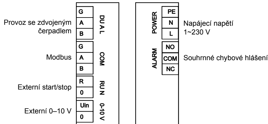
Obr. 9: Schéma zapojení Calio Z 30-60/-100, 32-80/-120, 40-80/-100 a 50-80
