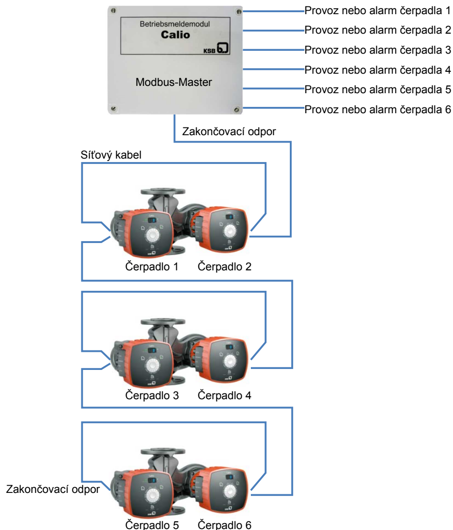
Obr. 11: Připojení čerpadel Calio Z k modulu provozních hlášení 01550860
