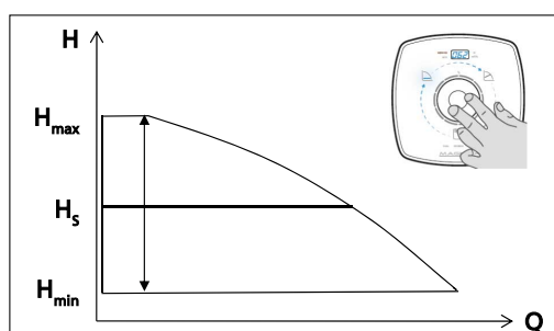
Obr. 17: Nastavení regulace na konstantní tlak
