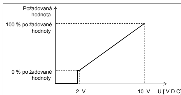
Obr. 27: Analogový signál 0–10 V jako zadání předepsané hodnoty na čerpadle
