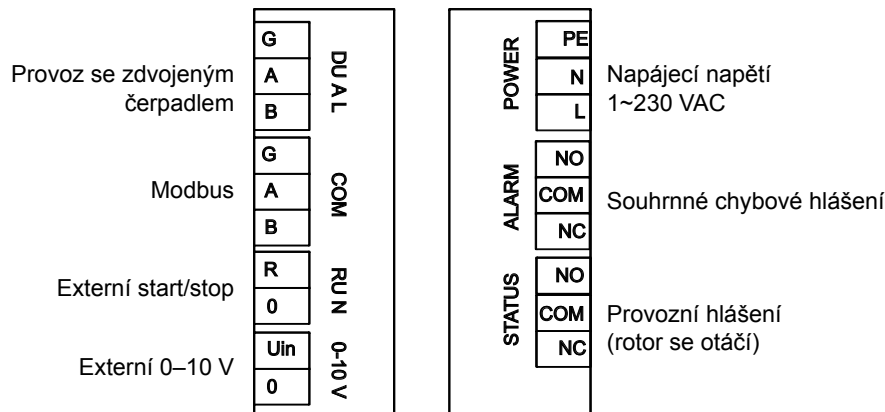
Obr. 10: Schéma zapojení Calio Z 40-120/-180, 50-100/-120 a 65-80/-120
