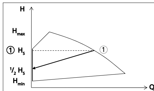
Obr. 19: Funkce Proporcionální regulace tlaku
