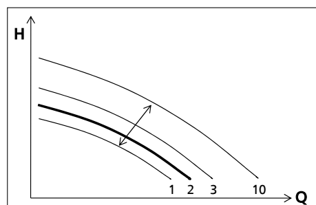
Obr. 22: Funkce Provoz s pevnými otáčkami
