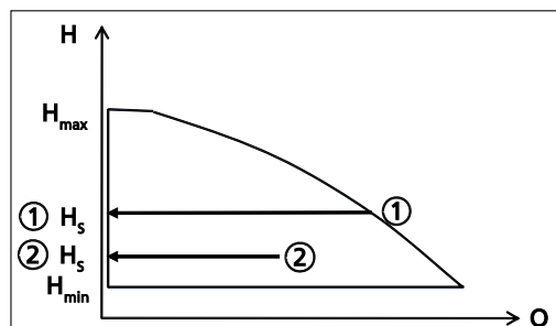
Obr. 16: Funkce Regulace na konstantní tlak
