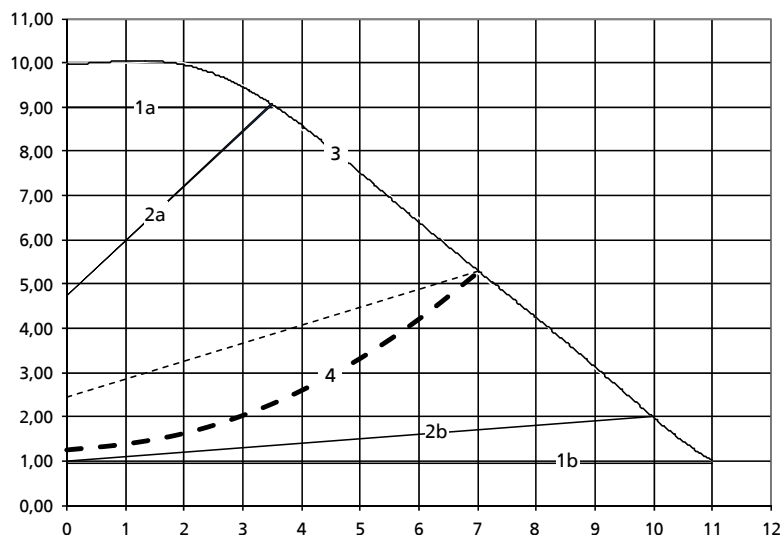
Obr. 25: Charakteristika režimu Eco-Mode na příkladu čerpadla konstrukční velikosti 25-10.0
