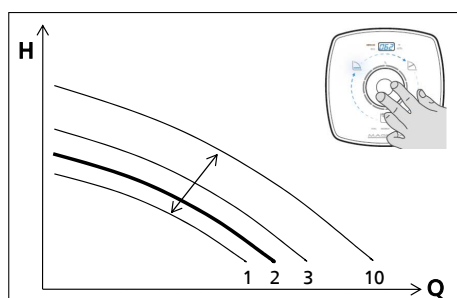
Obr. 23: Nastavení Provoz s pevnými otáčkami
