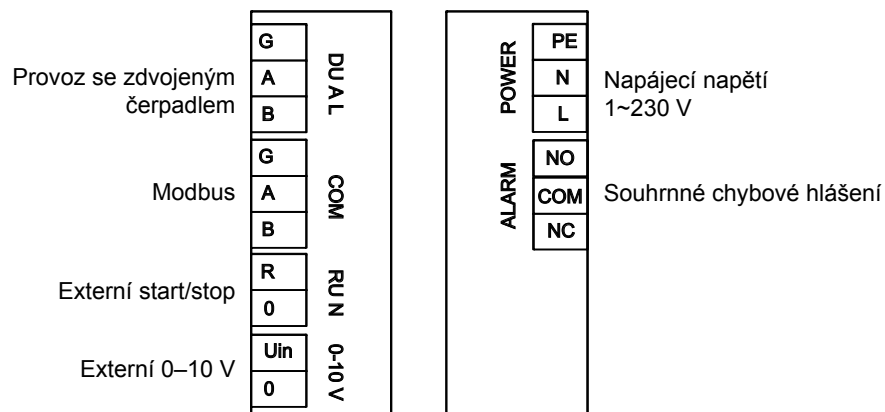
Obr. 35: Schéma elektrického zapojení typů Calio Z 30-60/-100, 32-80/-120, 40-80/-100 a 50-80
