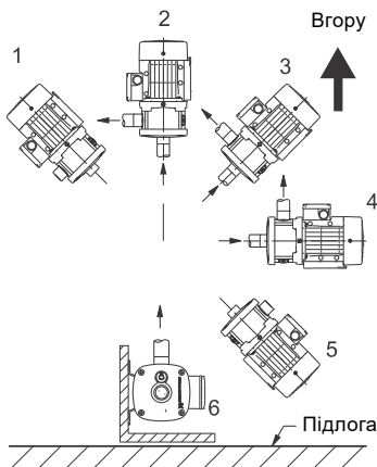
Рис. 1 Положення насоса
