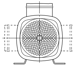
Рис. 6 Положення клемної коробки
