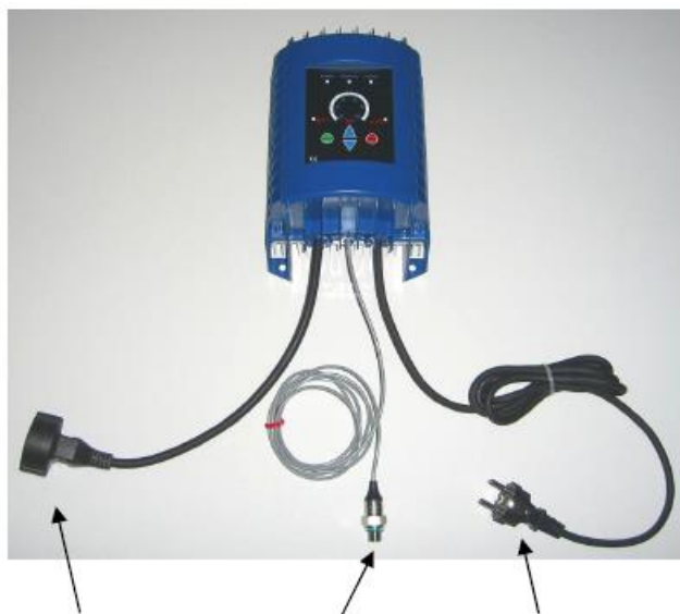
Obrázek 3: Připojení měniče
